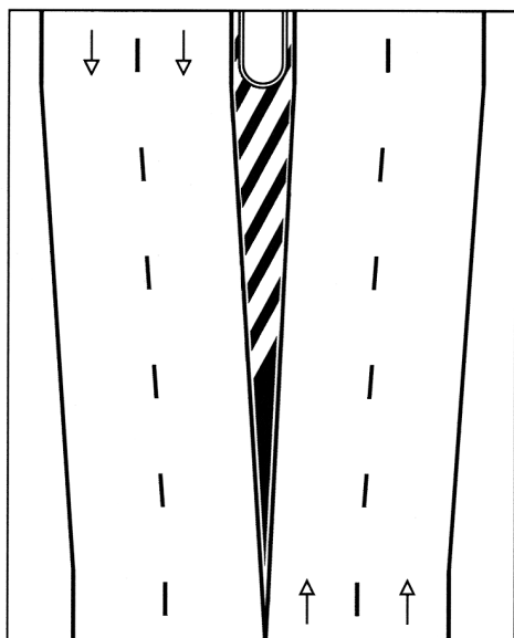
M17 – Raias obliquas delimitadas por linhas contínuas
